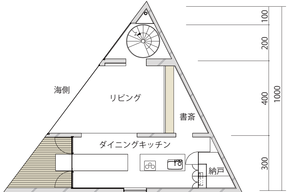
2階平面図
