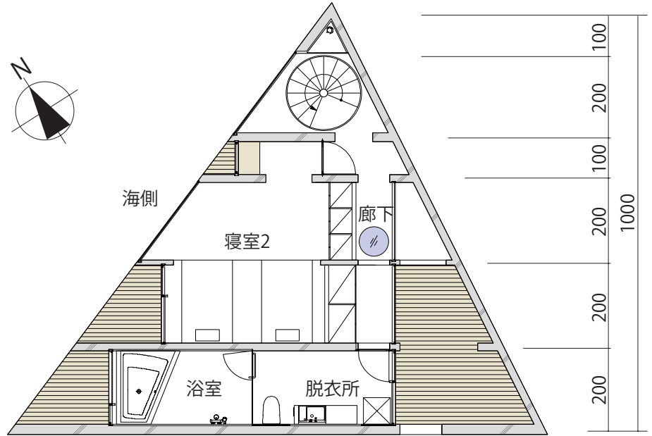
3階平面図
